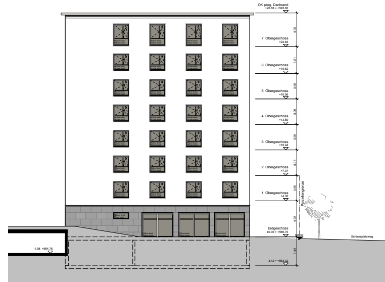
Ostfassade
