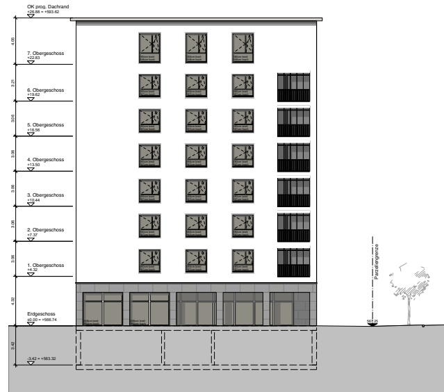
Nordfassade
