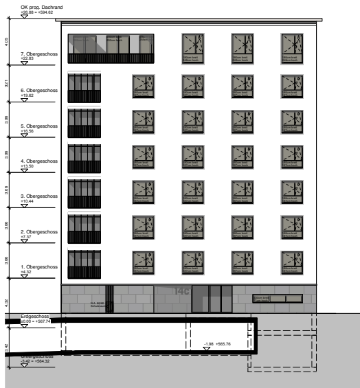
Südfassade
