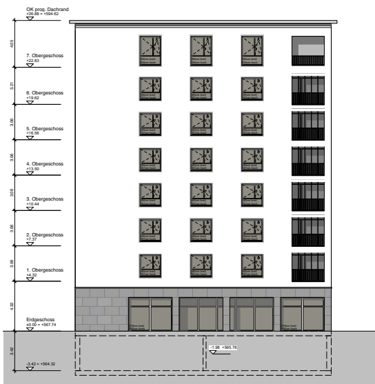
Nordfassade
