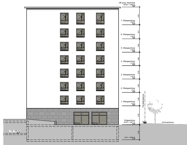
Ostfassade
