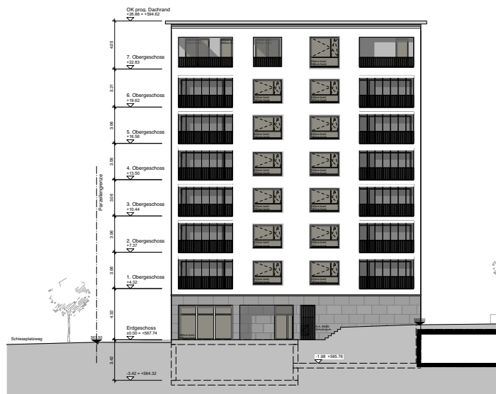
Westfassade
